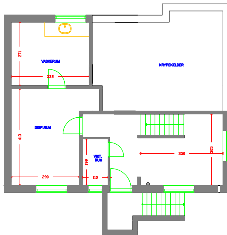
AFDELING 11 TYPE 22 2 RUMS 73 M2 KÆLDERPLAN
