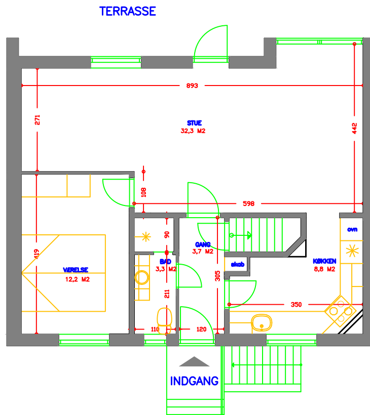
AFDELING 11 TYPE 22 2 RUMS 73 M2 STUEPLAN
