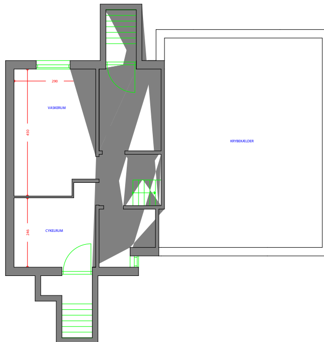
AFDELING 10 TYPE 46 4 RUMS 110 M2 KÆLDERPLAN
