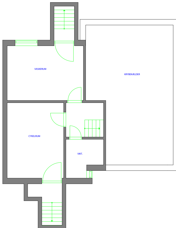
AFDELING 10 TYPE 33 3 RUMS 73 M2 KÆLDERPLAN
