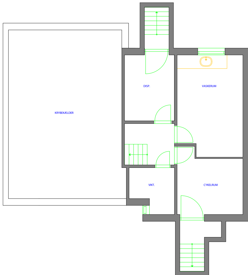
AFDELING 10 TYPE 32 3 RUMS 85 M2 KÆLDERPLAN
