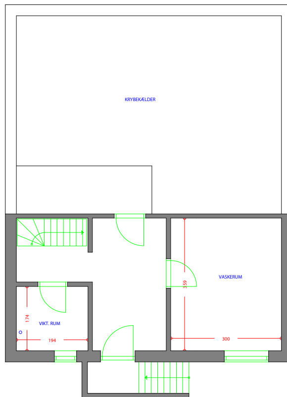
AFDELING 1 TYPE 23 2 RUMS 66M2 KÆLDERPLAN
