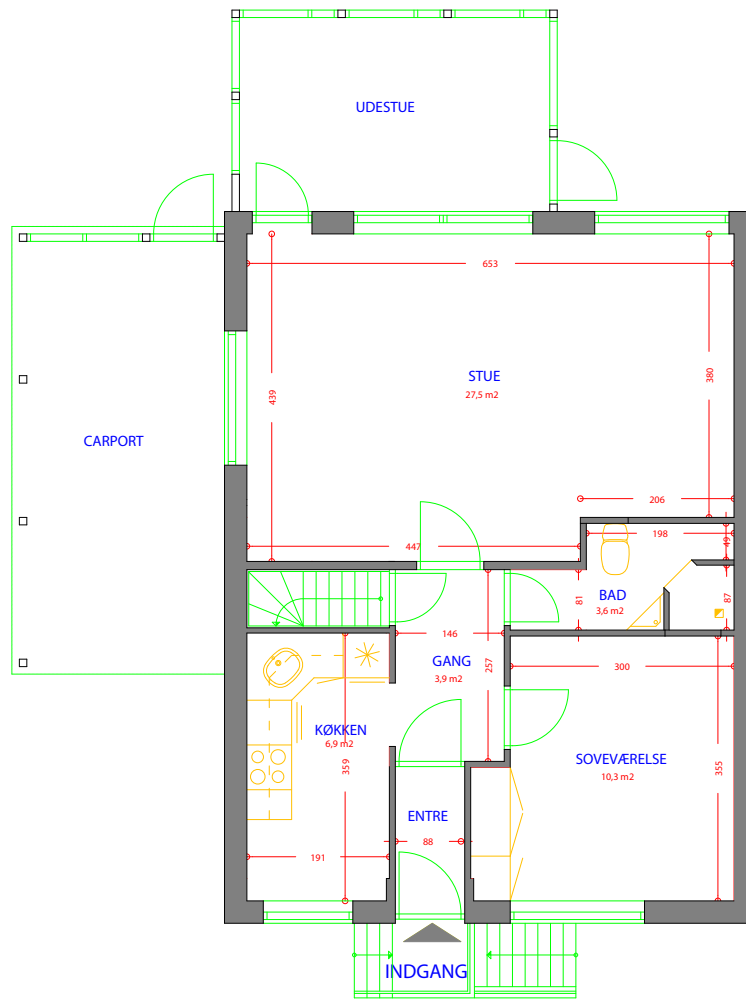
AFDELING 1 TYPE 23 2 RUMS 66M2 STUEPLAN
